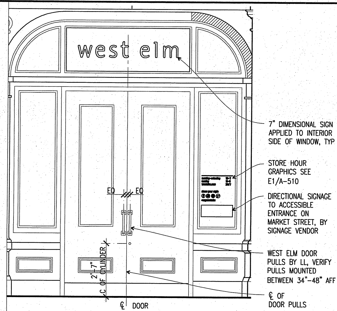
E5 ENTRY DOOR ELEVATION 3/8"=1'-0"
